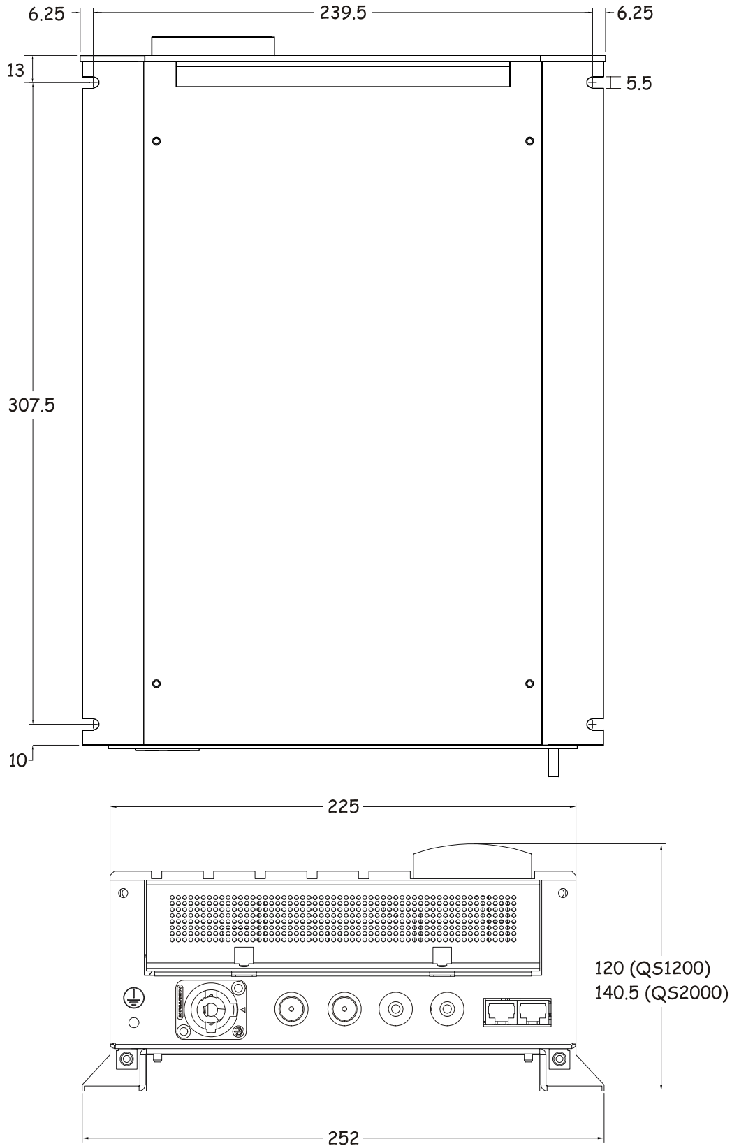
Figuur 7: afmetingen
